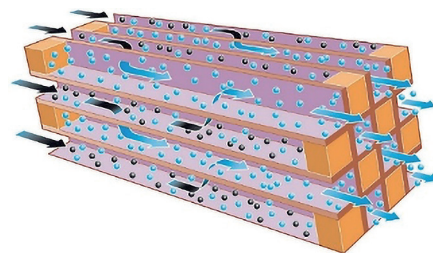
Schnitt durch den Dieselpartikelfilter
